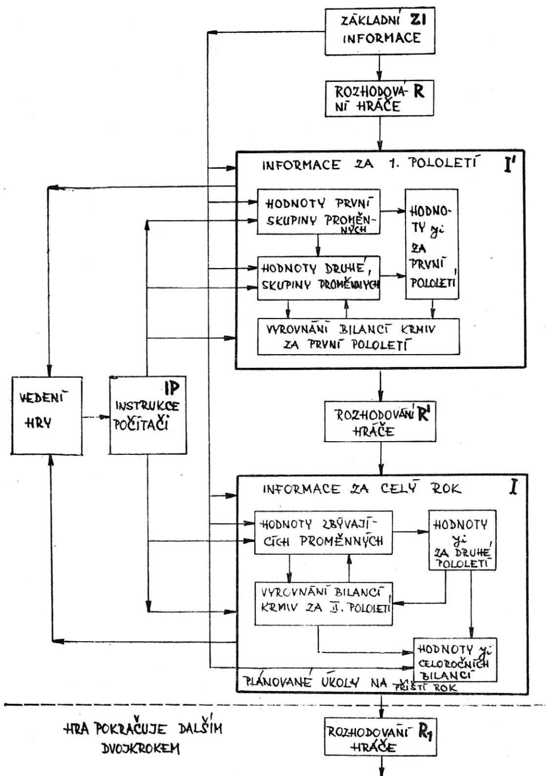
2. Funkční schéma hry
