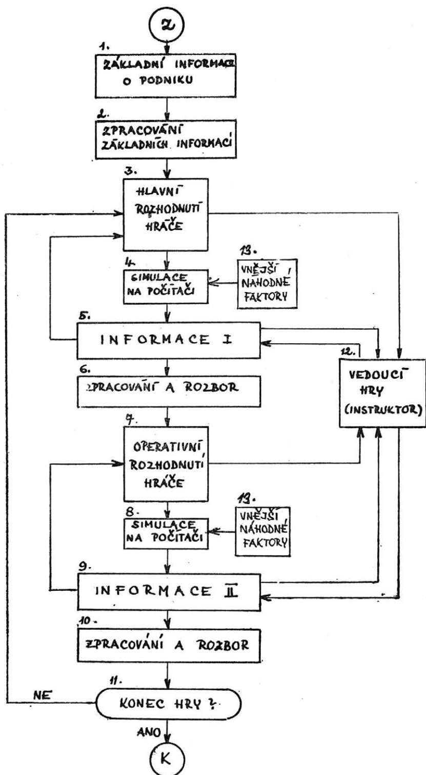
1. Schéma průběhu hry ZEMPO
